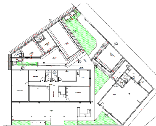
Figura 05 – Planta baixa da edificação do anexo cultural
